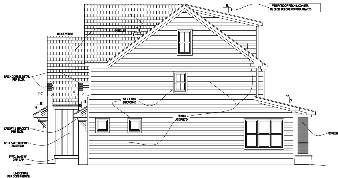
RIGHT ELEVATION
